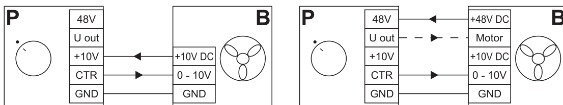
Schaltplan
