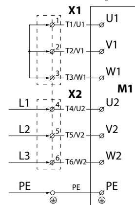
Anschlusschema für einen Ventilator mit einem zweistufigen Motor
