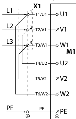
Anschlusschema für einen Ventilator mit einem einstufigen Motor
