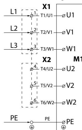
Anschlusschema für einen Ventilator mit einem zweistufigen Motor
