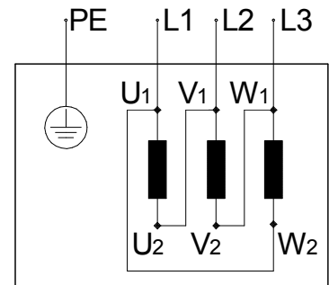
Anschlußplan Drehstrommotor 400/690 V
