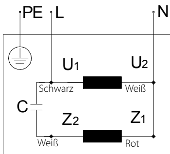
Anschlußplan Einphasenmotor 230 V
