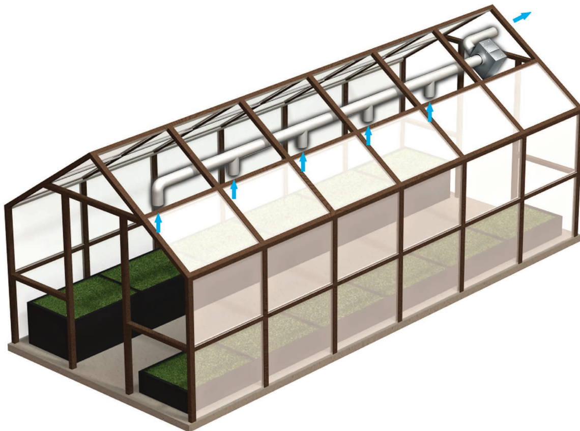
KSA fan greenhouse ventilation example
