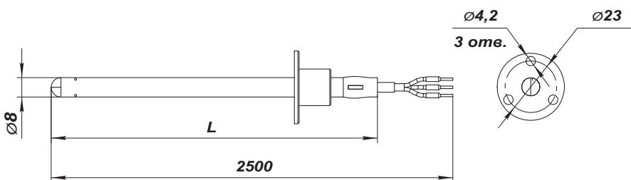
Канальный датчик температуры КДТ2-М
