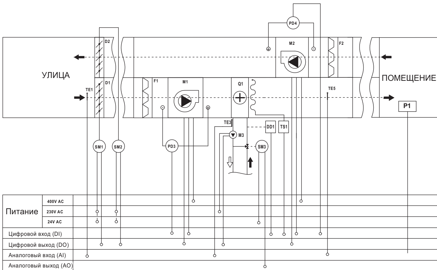
Приточно-вытяжная установка (АС/ЕС двигатель) с жидкостным воздушонагревателем
