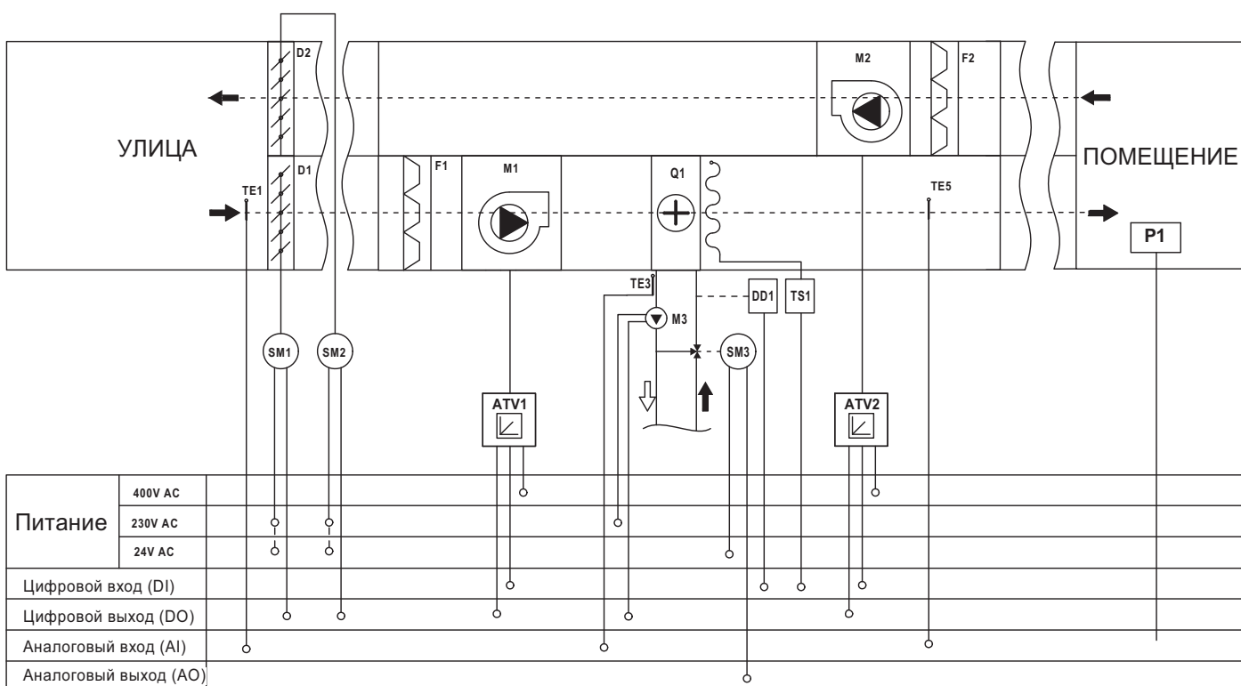
Приточно-вытяжная установка (АС двигатель с частотным преобразователем/ ЕС двигатель) с жидкостным воздушонагревателем
