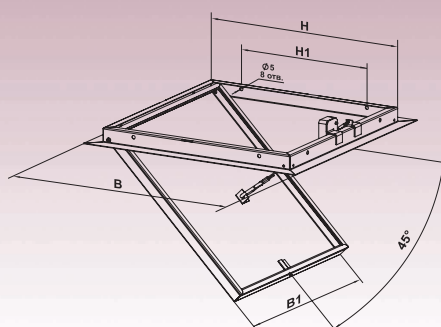
Ревизионные металлические дверцы для потолочного монтажа
