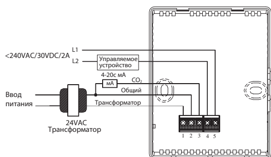
Рис. 4. Схема подключения
