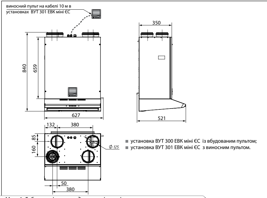
Мал. 1. Габаритні та приєднувальні розміри установки з витяжкою
