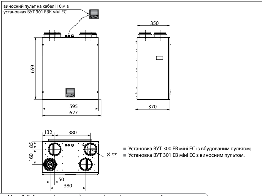
Мал. 2. Габаритні та приєднувальні розміри установки без витяжки
