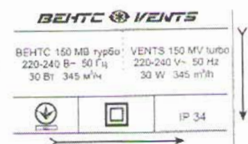
150 MV turbo
