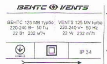
125 MV turbo
