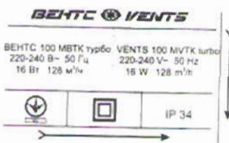
100 MBTK turbo
