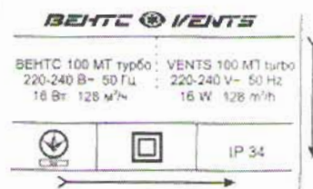
100 MT turbo
