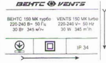
150 MK turbo
