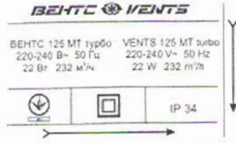
125 MT turbo
