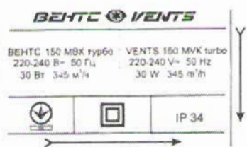
150 MBK turbo
