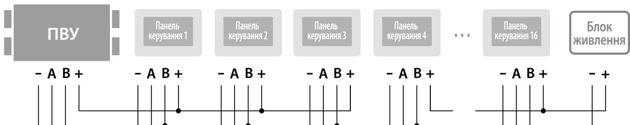
Приклад 2 У разі підключення більше 3 панелей до однієї ПВУ необхідно використовувати зовнішнє джерело живлення.
