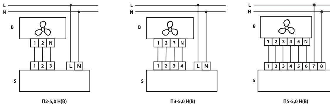
Варіанти підключення перемикача
