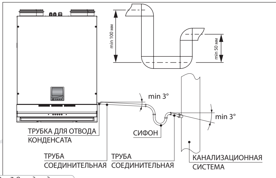
Рис. 7. Отвод конденсата
