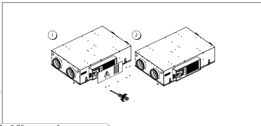
Рис. 9. Обслуживание блока управления
