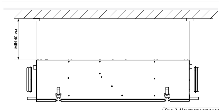
Рис. 3. Монтаж установки
