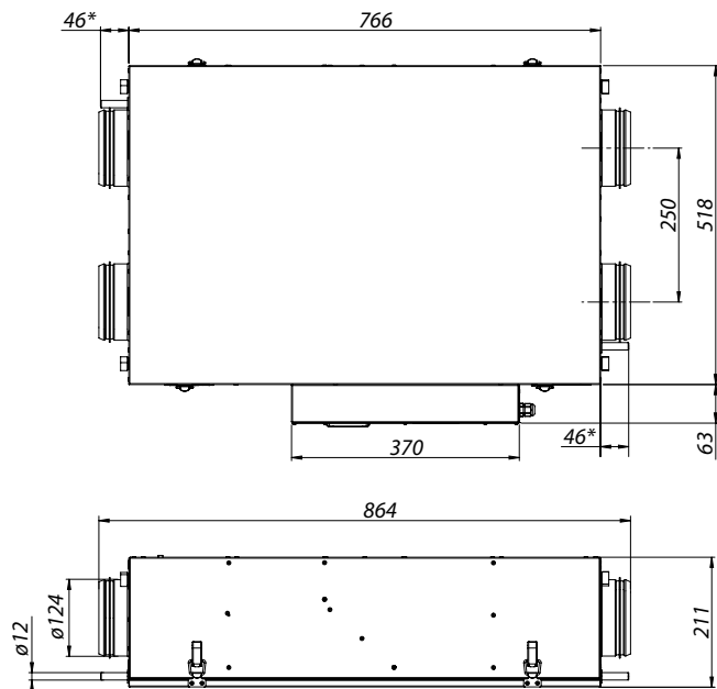
Рис. 1. Габаритные и присоединительные размеры установки
