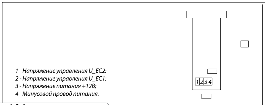
Рис. 6. Вид пульта со стороны разъема
