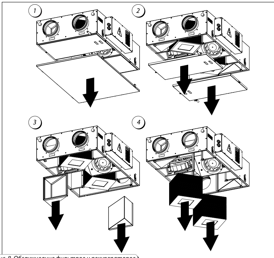
Рис. 8. Обслуживание фильтров и рекуператоров
