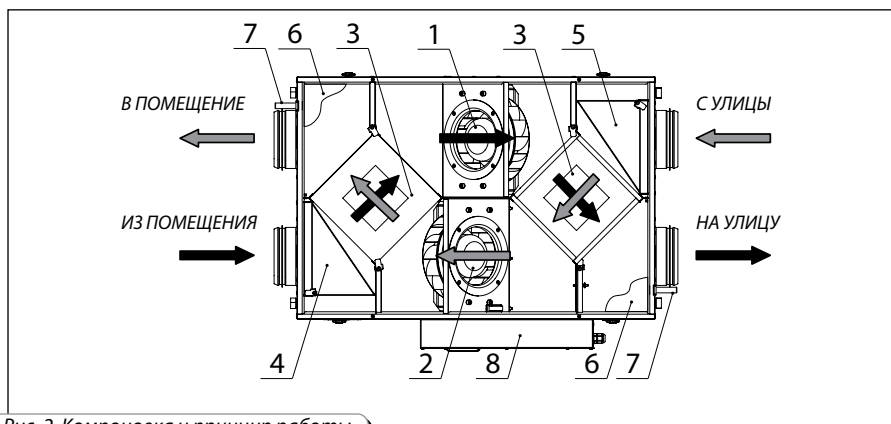
Рис. 2. Компонновка и принцип работы
