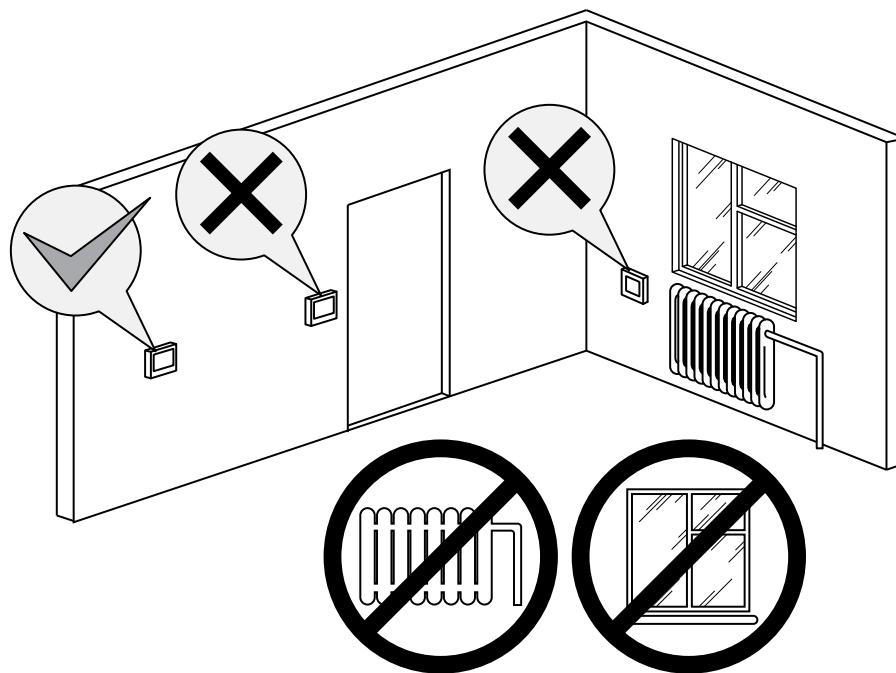
Abb. 5. Montage des digitalen Thermostats.
