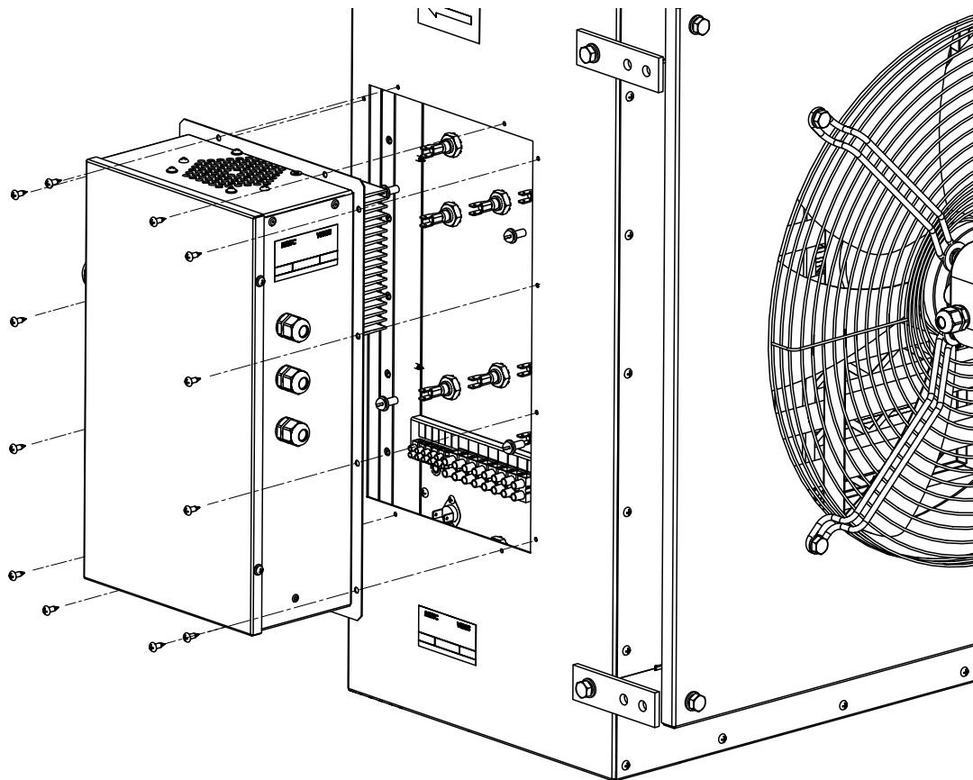
Abb. 3. Montage der Steuereinheit
