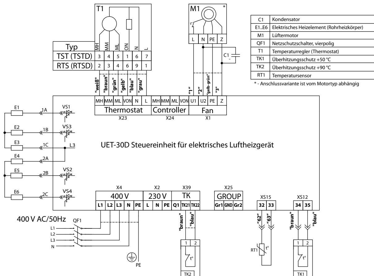
Abb. 8. Anschlußschaltplan für UET-30D (Schutzschalter)
