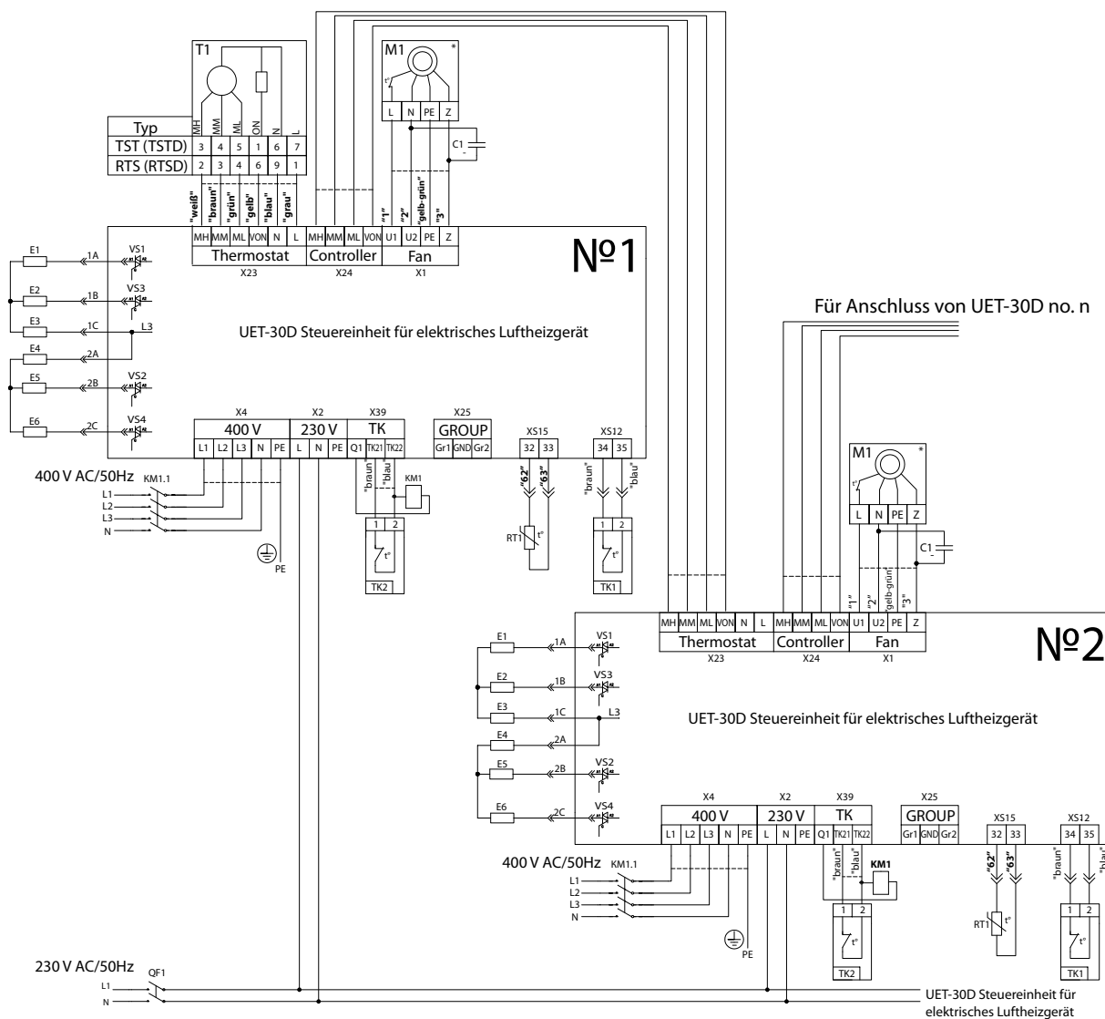
Abb. 11. Anschlussplan für mehrere Steuereinheiten UET-30D
