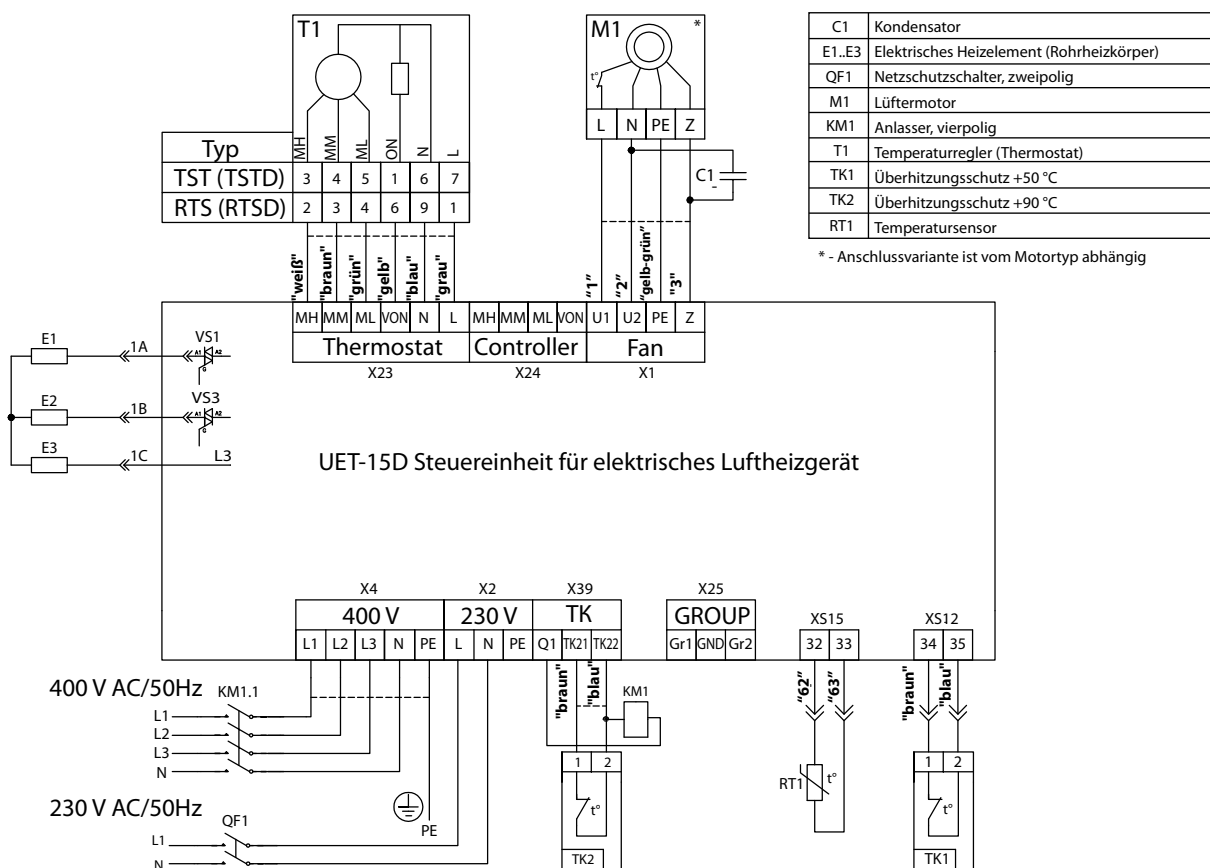
Abb. 7. Anschlußschaltplan für UET-15D (Magnetanlasser)
