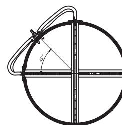
МВП 355-630
